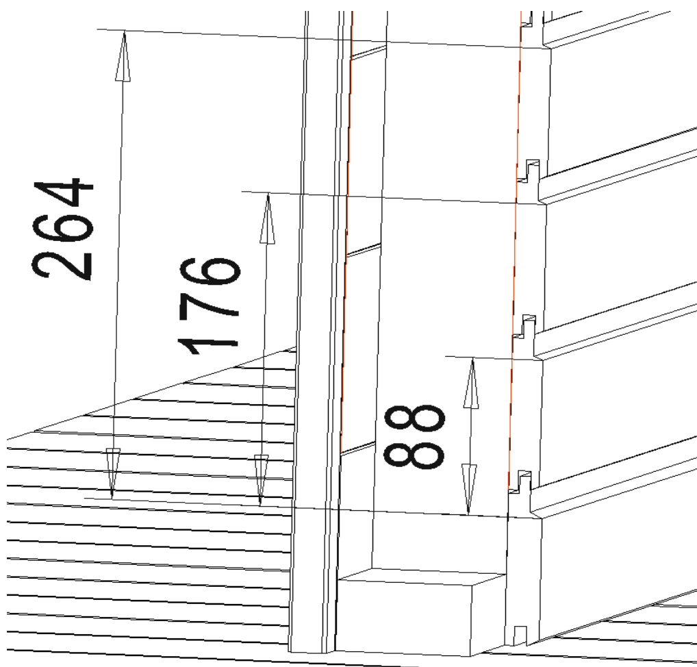
27. Sisäpaneelin paneelijako
