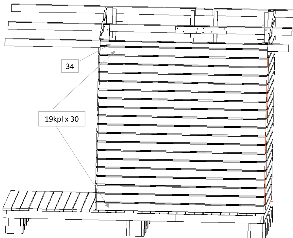
16. Asenna paneeli oviseinään, muista paneelijako.
