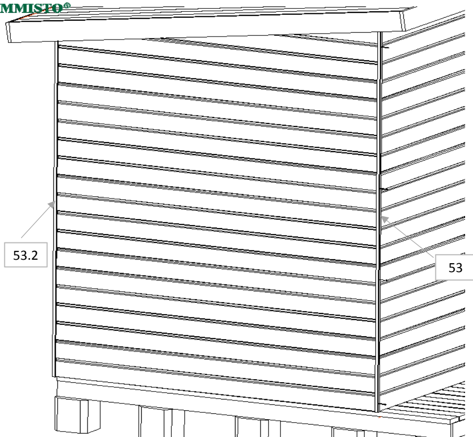
26. Asenna rimat saunan nurkkiin 2,1 x 50 nauiloilla
