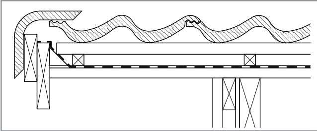
Päätyreunatiili.
