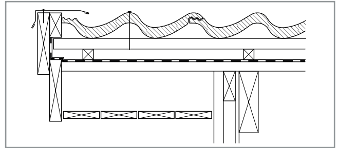
Päätyräystäspelti.
