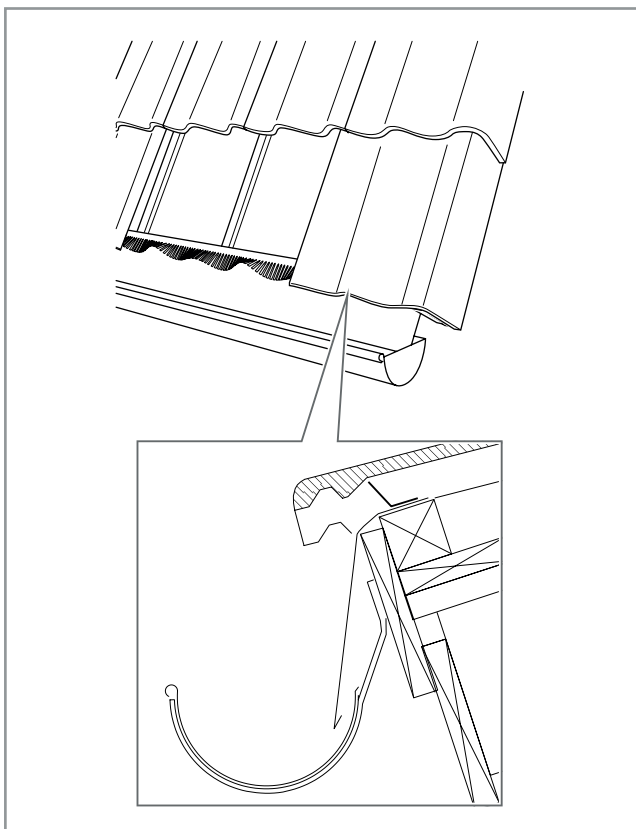
Lintuesteen asentaminen.
