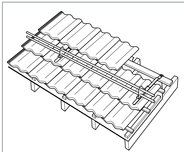
Lumiesteen asentaminen.
