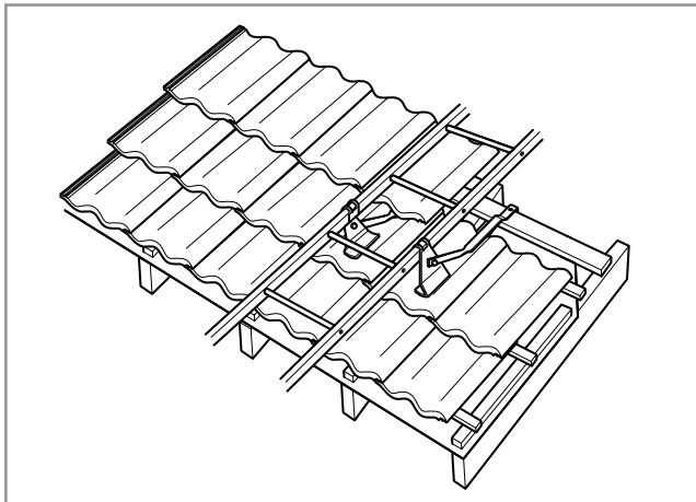
Lapetikkaiden asentaminen.
