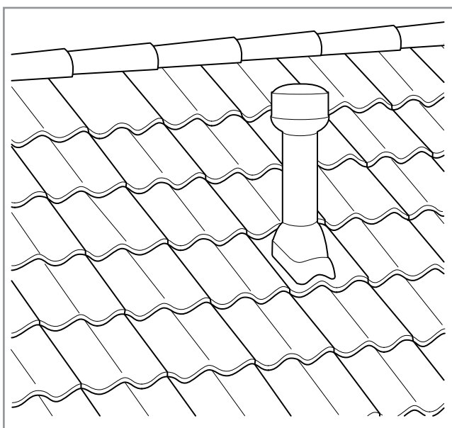
Ilmanvaihtoputki asennettuna.
