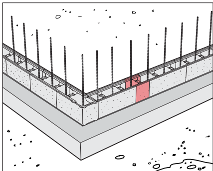
Kuva 12. Harkkoseinän rauditusperiaate.
