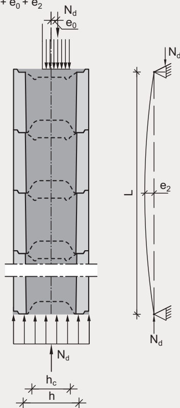
Kuva 3. Seinän staattinen malli ja pystykuorman epäkeskisyyden laskenta.
