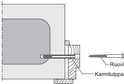
Kuva 15. Puukarmin kiinnityisperiaate kulmaharkkoon.
