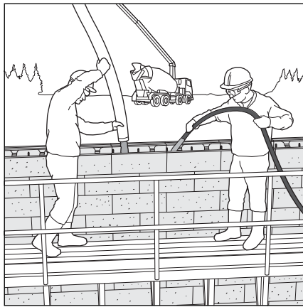
Kuva 14. Harkkoseinän betonointi.
