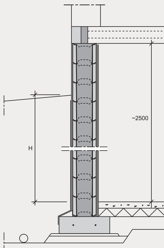
Kuva 2. Maanpaineeseinä
