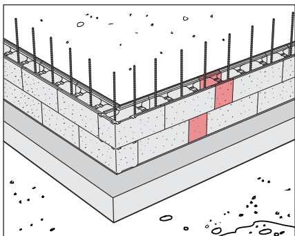
Kuva 11. Sovitepalojen sijoittelu harkkoseinässä.
