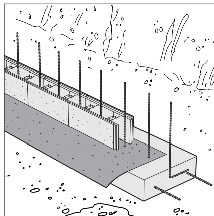
Kuva 8. Ensimmäinen harkkokerros.
