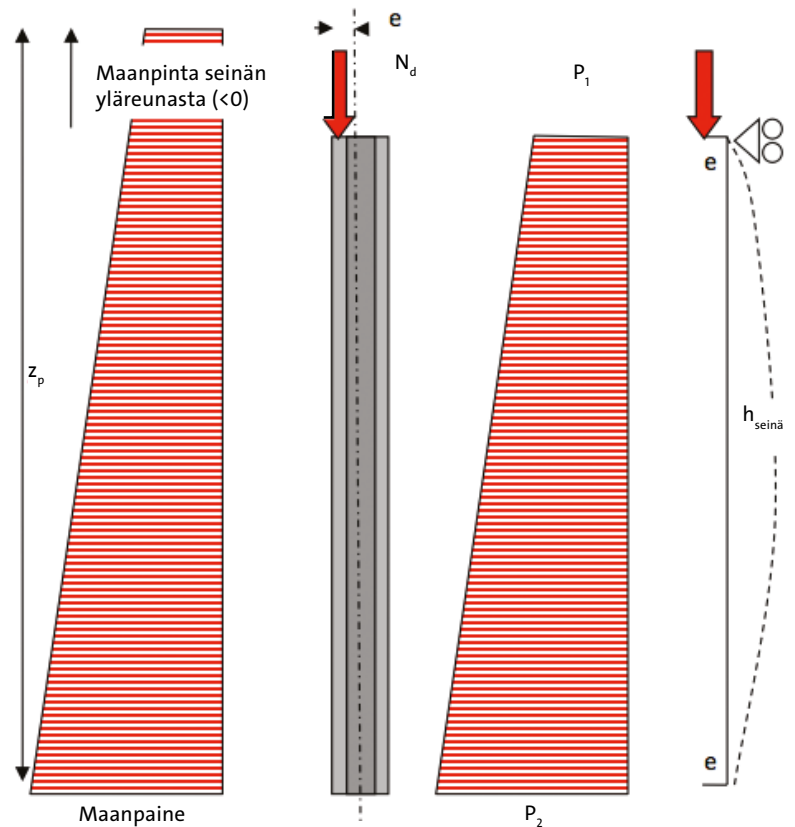
Kuva 4. Maanpaine, kun seinän yläreuna on maanpinnan alapuolella.
