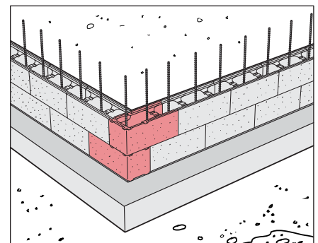
Kuva 9. Ladottaessa kulmaharkkojen välille syntyvä nurkkalukitus.
