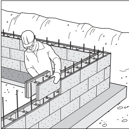
Kuva 10. Ladottaessa harkkojen ympäröintiponttauksen ansiosta harkkomuurista tulee jo ladottaessa tukeva ja vakaa.
