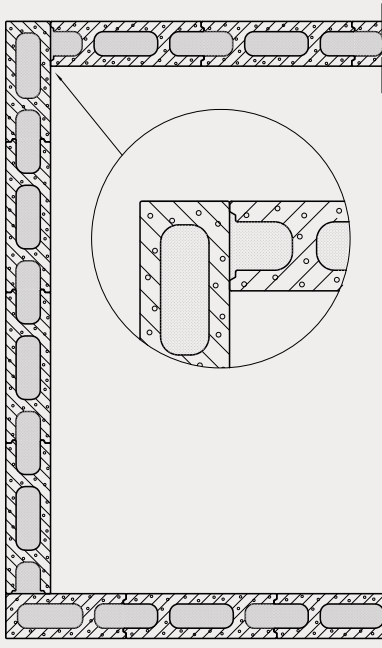
Kuva 1. 150 mm ja 200 mm leveiden Leca-valuharkkojen ladontaperiaate.
