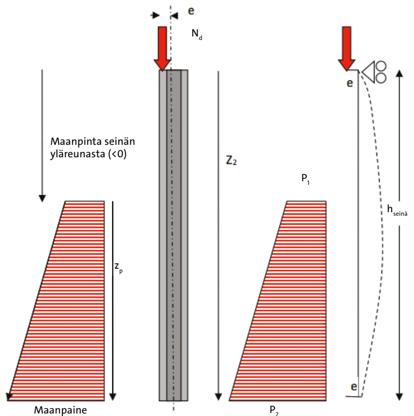
Kuva 5. Maanpaine, kun seinän yläreuna on maanpinnan yläpuolella.
