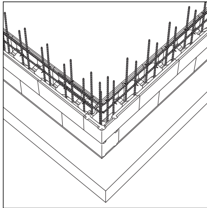
Kuva 12. Harkkoseinän rauditusperiaate.
