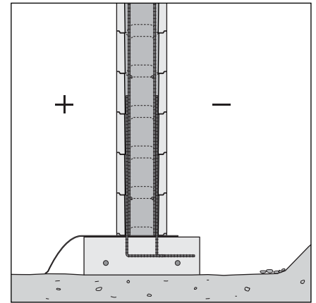
Kuva 13. Harkkoseinän rauditusperiaate.
