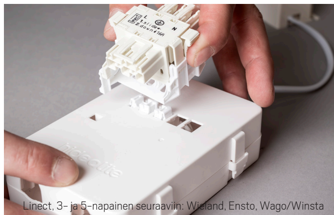
Ruuviton vedonpoisto kaapelille tai taipuisalle suojaputkelle 16mm
