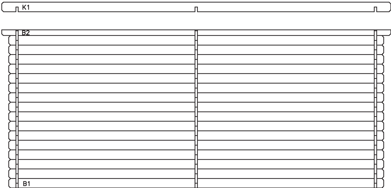
Lillevilla Unnukka: 5100 x 3000 mm
