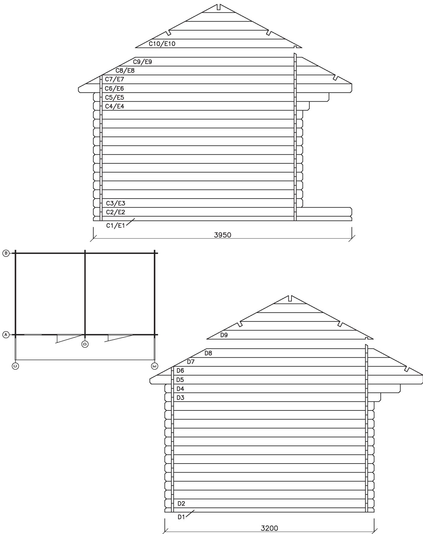
Lillevilla Unnukka: 5100 x 3000 mm
