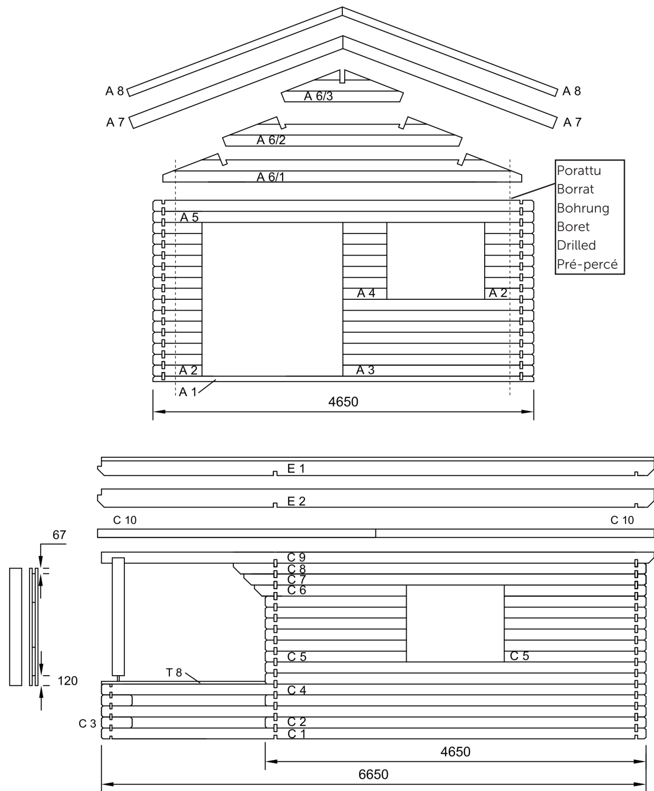
Lillevilla Saimaa: 4450 x 4450 mm
