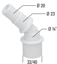
LVI 248 8936 Tuotenro 78610
