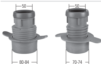
2½" valurautamuhvi 83009
