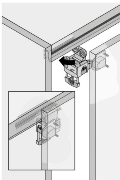
Ovien kiinnitys
