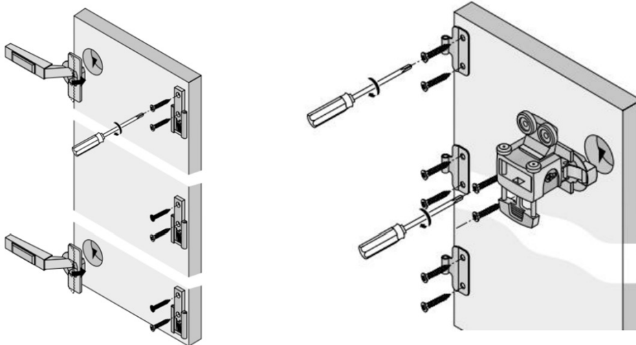
Saranoiden kiinnitys
