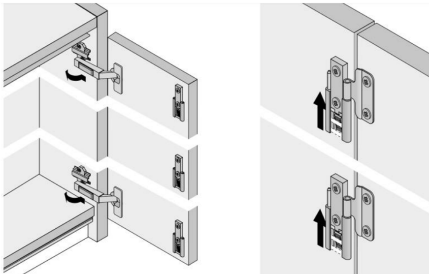
Ovien kiinnitys
