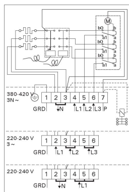
Electrical connections of BC heater Elektroanslutningar av Saunaofens BC
