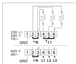
Electrical connections of BC-E heater Elektroanslutningar av Saunaofens BC-E
