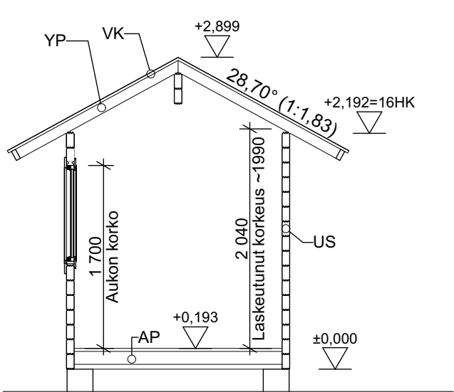
Leikkaus A-A
