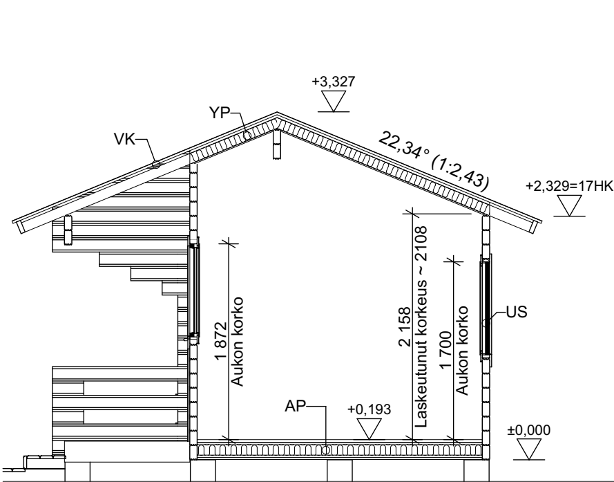
Leikkaus A-A
