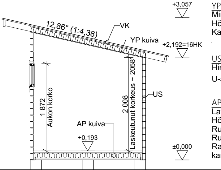
Leikkaus A-A
