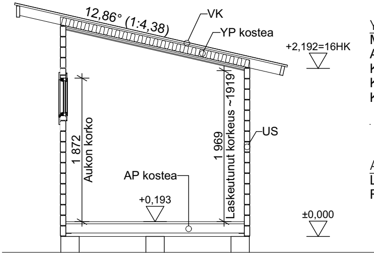
Leikkaus B-B
