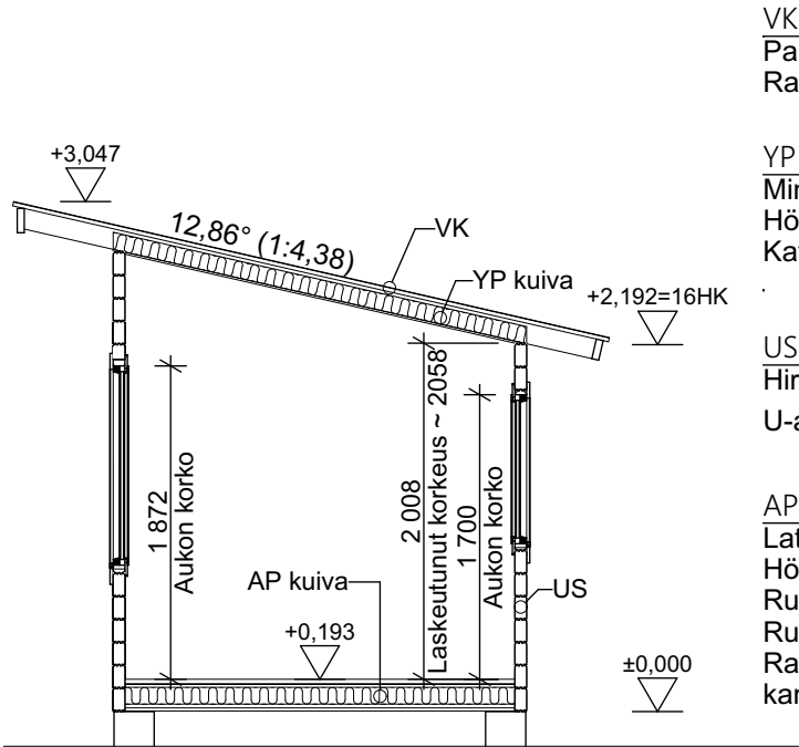
Leikkaus A-A
