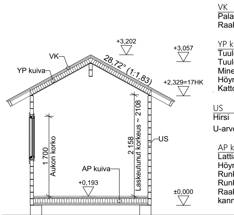
Leikkaus A-A
