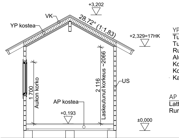
Leikkaus B-B
