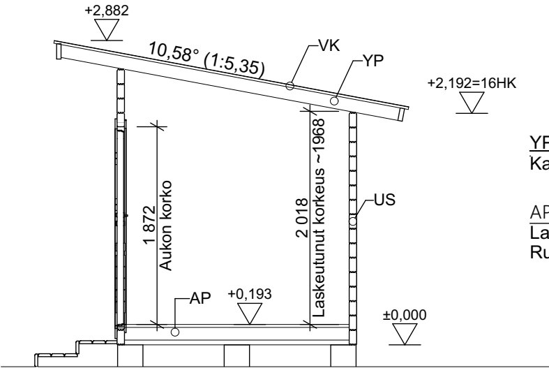
Leikkaus B-B
