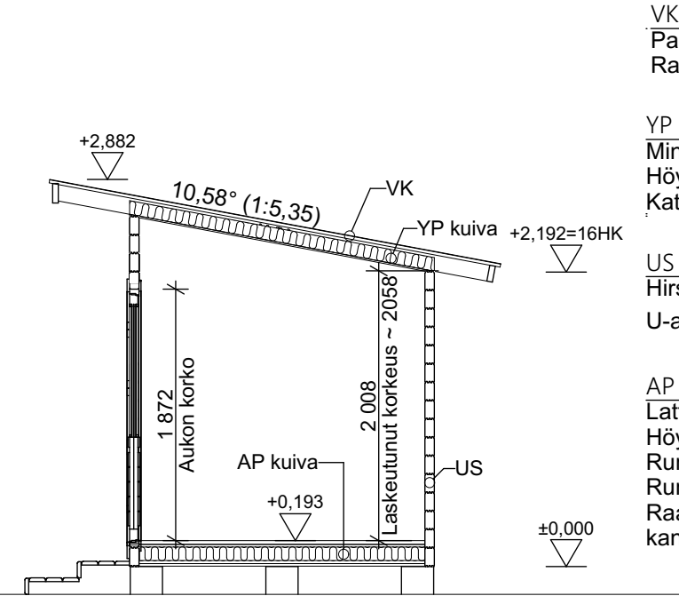
Leikkaus A-A
