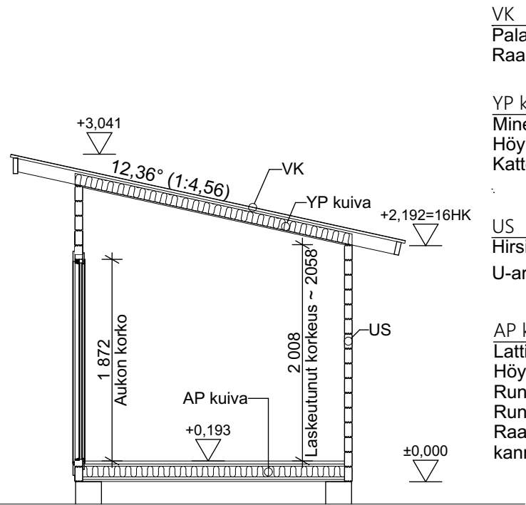
Leikkaus A-A
