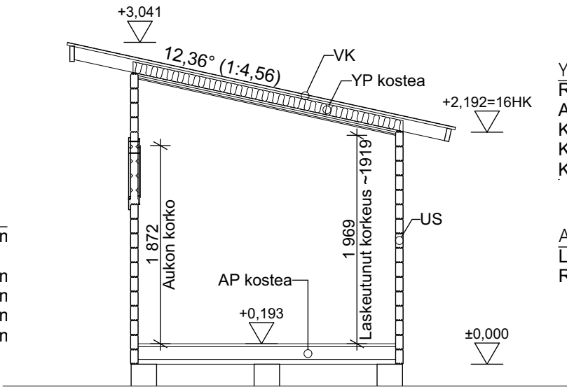
Leikkaus B-B
