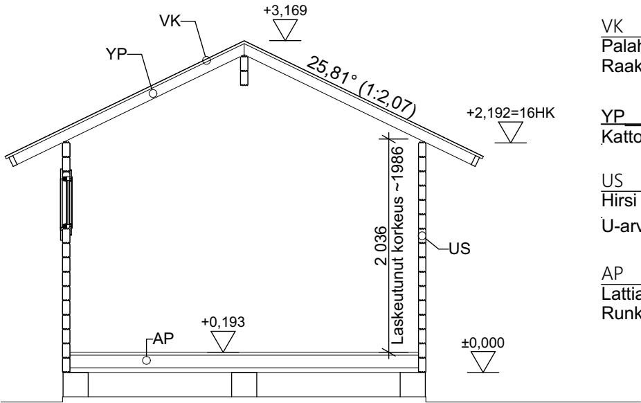
Leikkaus A-A
