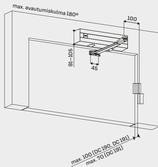
Sulkeutumispuoli
