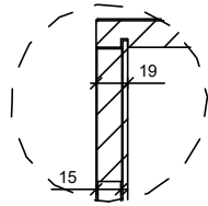
DET1 1:5
