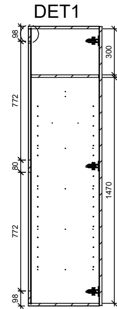
A-A
