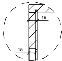
DET1 1:5
