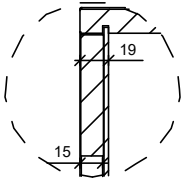
DET1 1:5
