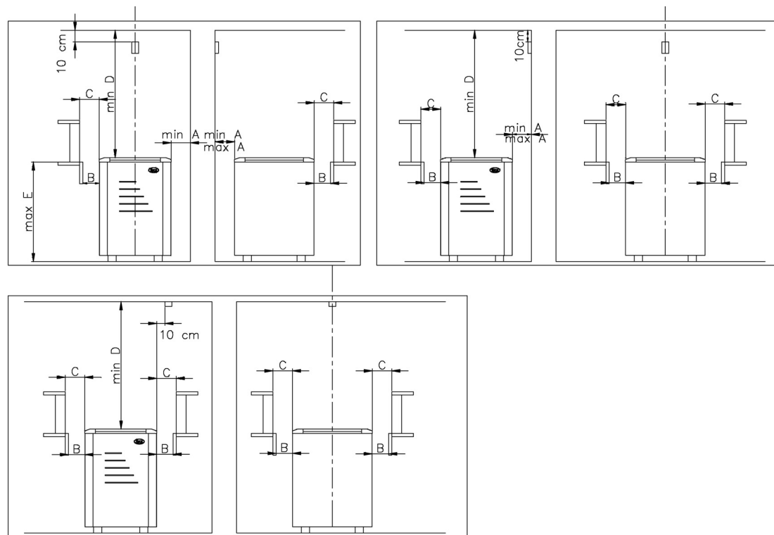
Joonis 2. T-2003 ja B-2003 andurikarbi paigaldamine.
