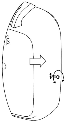
5 paveikslėlis. Valdymo pulto dangtelio nuėmimas.
