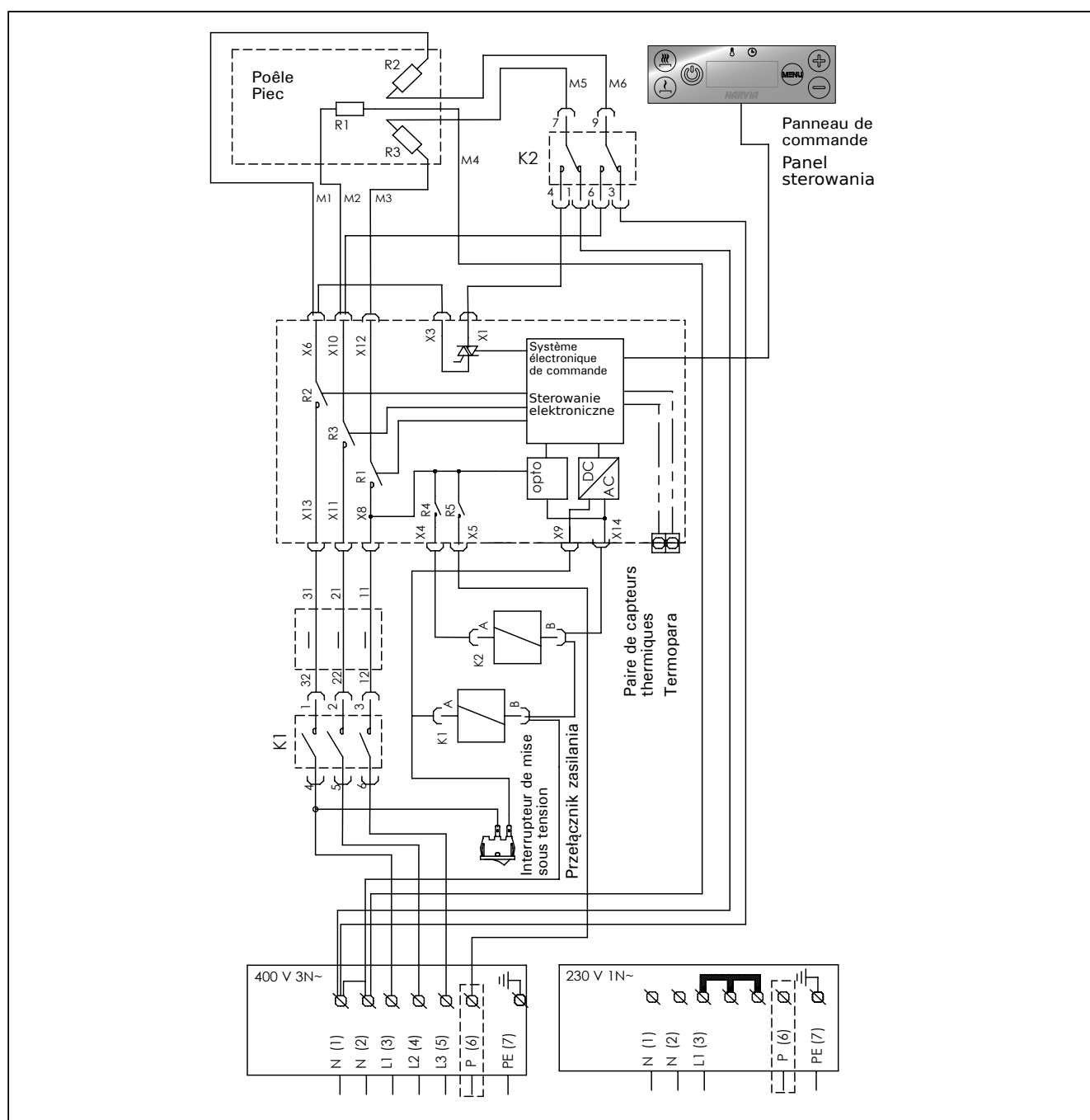
Figure 12. Connexions électriques des poêles Rysunek 12. Połączenia elektryczne pieca
