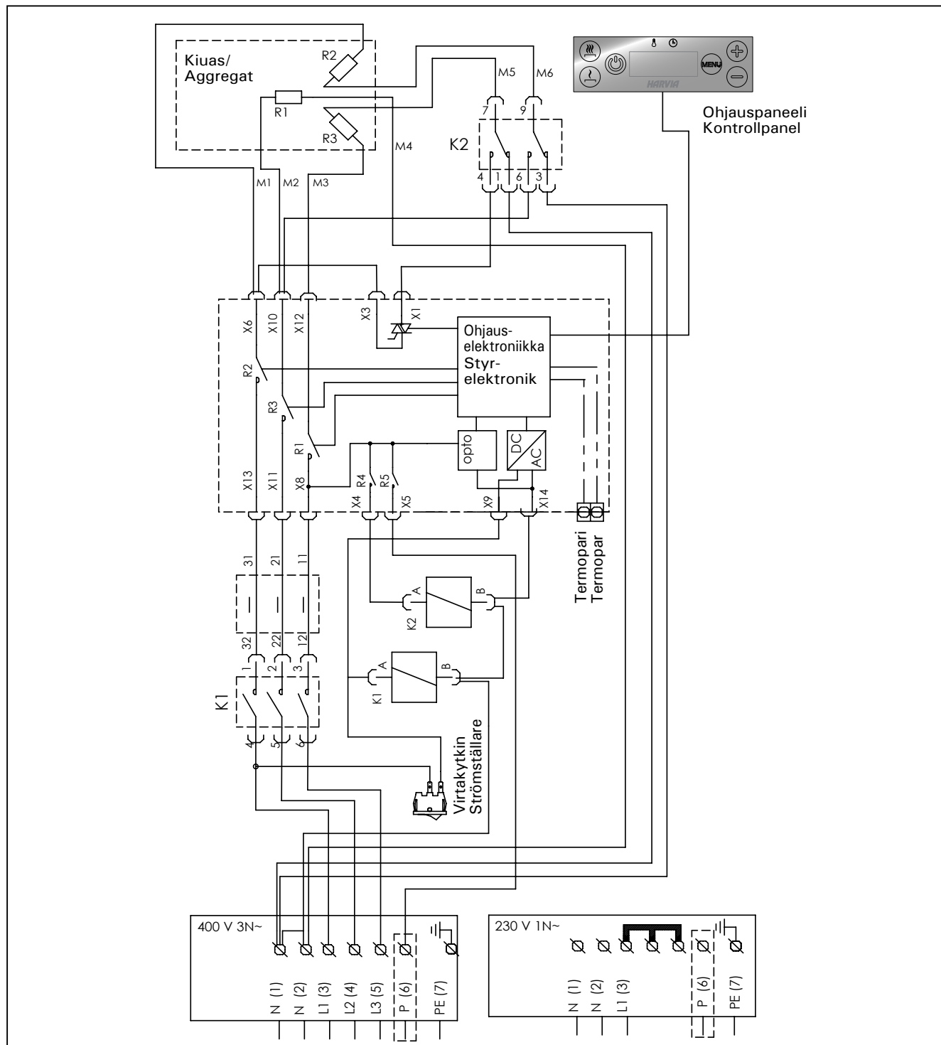
Kuva 12. Kiukaan sähkökytkennät
