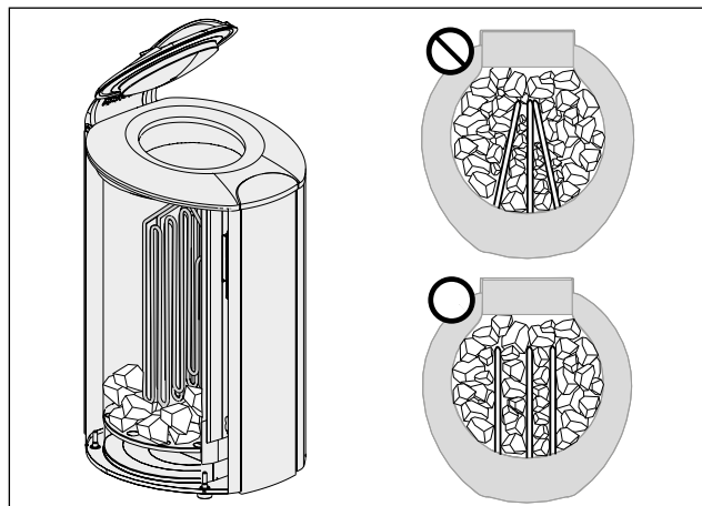
Kuva 5. Vastuksien tukeminen. Bild 5. Support av elementer.
