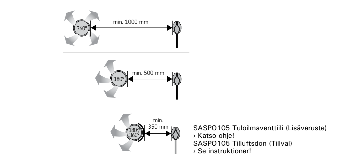
Kuva 4. Tuloilmaventtiilin vähimmäisetäisyys lämpötila-anturiin.
