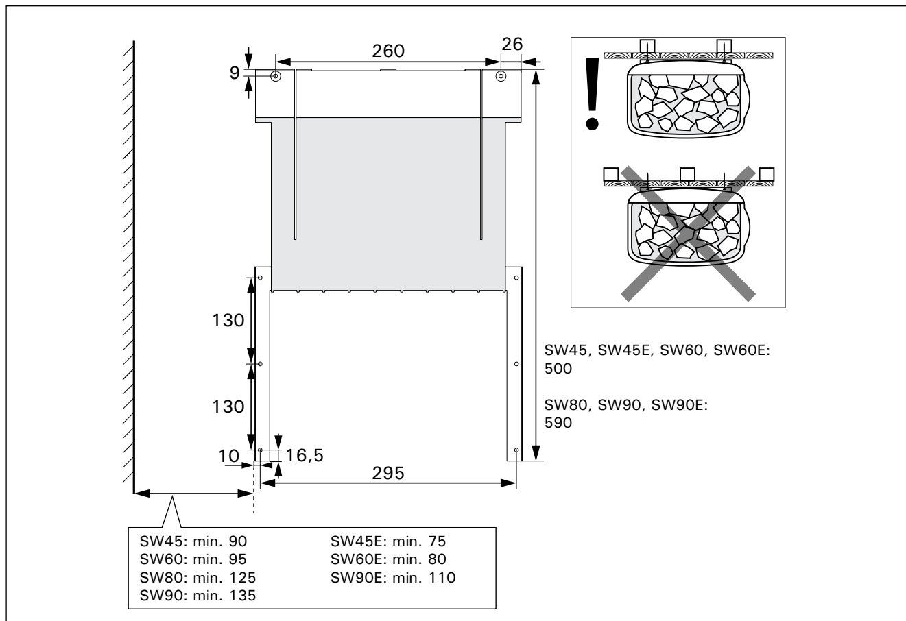
Figure 7. Support mural, dimensions en millimètres
