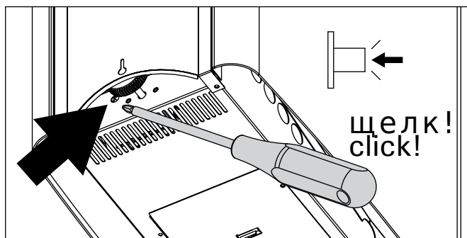
Рисунок 12. Восстановление рабочего состояния после срабатывания режима защиты от перегрева Joonis 12. Ülekuumenemiskaitse tagastamine
