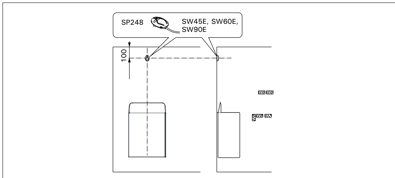
Figure 6. Installation du capteur (toutes les dimensions sont fournies en millimètres)
