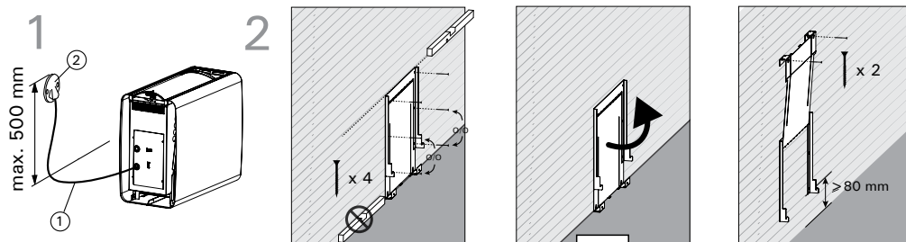
Figura 7. Montaggio a parete (Tutte le dimensioni sono in millimetri)
