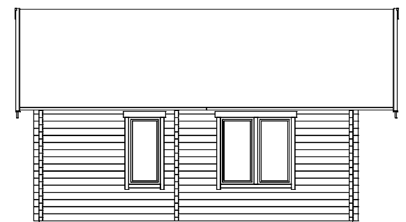
Pohja, leikkaus- ja julkisivupiirustukset suhteessa M 1:100
