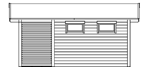
Pohja, leikkaus- ja julkisivupiirustukset suhteessa M 1:100
