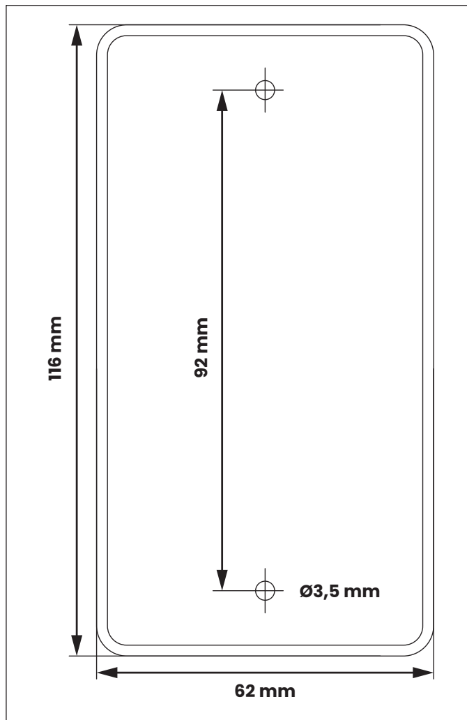
Hälytyspaneelin asennusmitat
