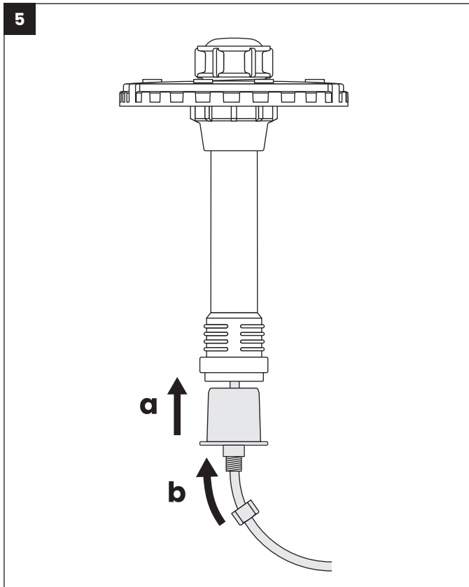
Kuva 5. Aseta piirikortti suojauputken (3) sisään. Vaihe a: paina päätytulppa (2) suojauputken (3) muhvin pohjaan asti. Vaihe b: kiristä kaapeliläpivienti (1).
