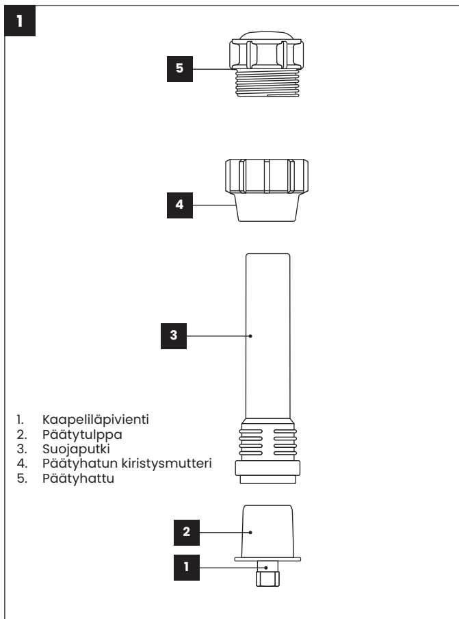
Kuva 1. Lähetinyksikön osat.
