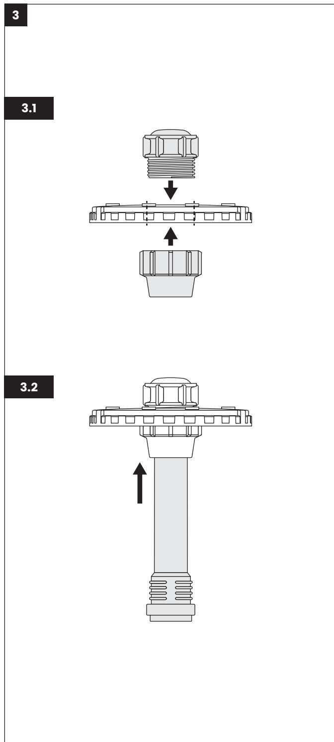
Kuva 3. Asenna päätyhattu (5) reikään ja kiinnitä se sen kiristysmutterilla (4) niin, että muhvi osoittaa säiliön sisään päin (kuva 3.1). Paina suojaputki (3) päätyhatun muhvin pohjaan asti (kuva 3.2).
