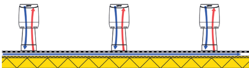
Alipain ainutlaatuisen rakenteen ansiosta ilmaa virtaa enemmän.
