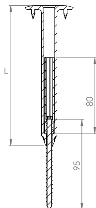
VILPE Croco A -kiinnike + Croco säädettävä ruuvi 95. L on Croco-mallin pituus.
