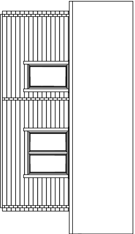
JULKISIVU 2
