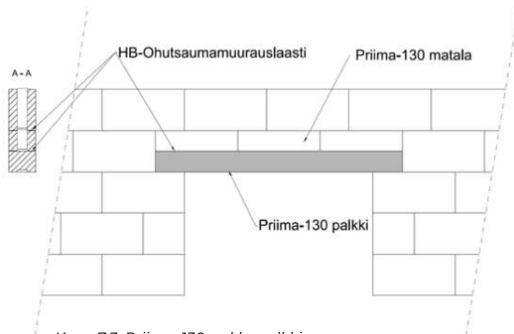
Kuva 7.3. Priima-130 aukkopalkki.
