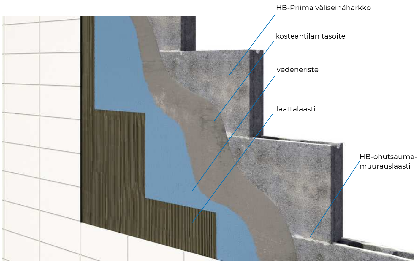
Kuva 8. Rakenneleikkaus.
