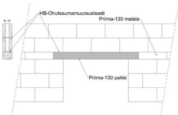
Kuva 7.4. Priima-130 aukkopalkki.
