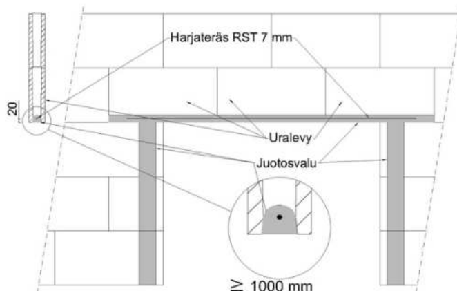
Kuva 7.1. Aukonylitys uraharkkoilla.
