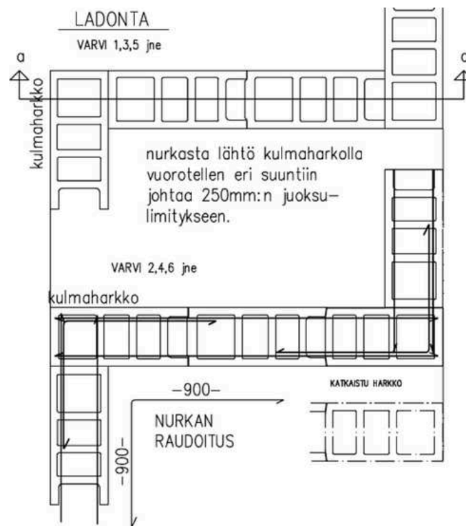
Kuva 6. Nurkkaladonna periaate.
