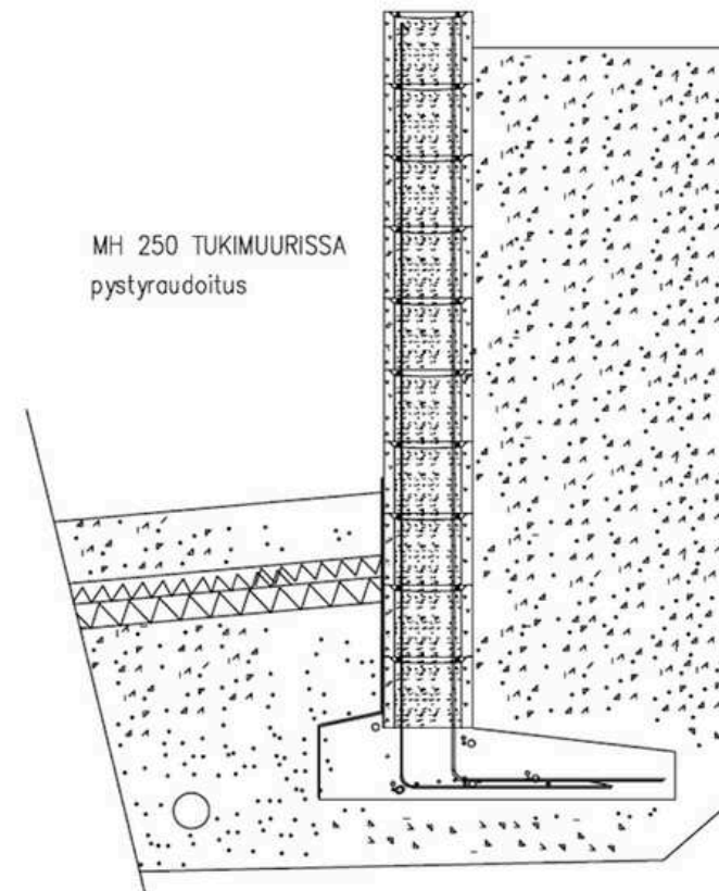
Kuva 14. Tukimuuuri.
