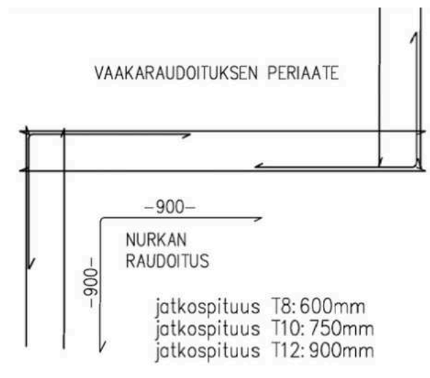
Kuva 7. Vaakaraudoituksen periaate.
