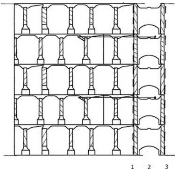
Kuva 9. Muottiharkkojen pystyleikkaus.
