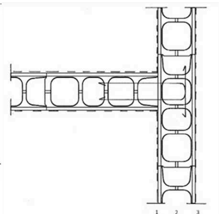
1 Tasoite 5 mm 2 VALU-200 harkko betonivalu ja raudoitu rakennesuunn. ohj. mukaan 3 Tasoite 5 mm
