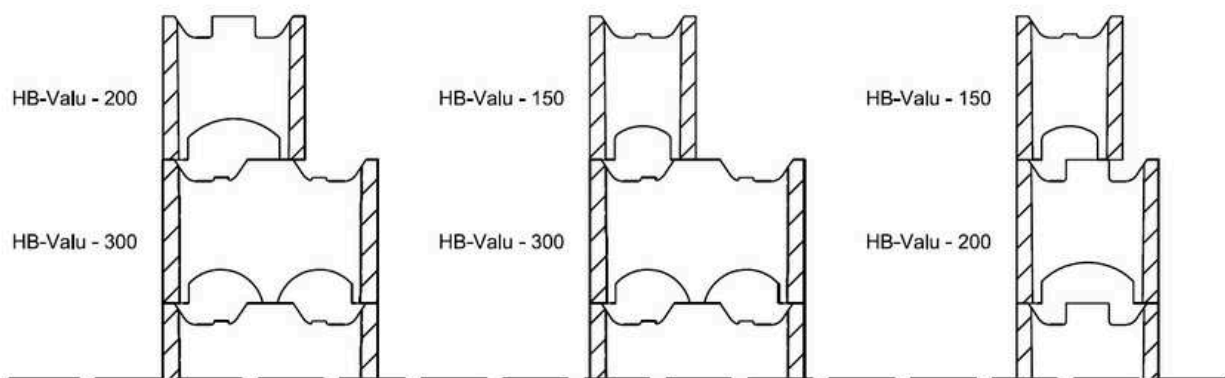
Kuva 17. Perustusten yläpään kavennusvaihtoehdot.
