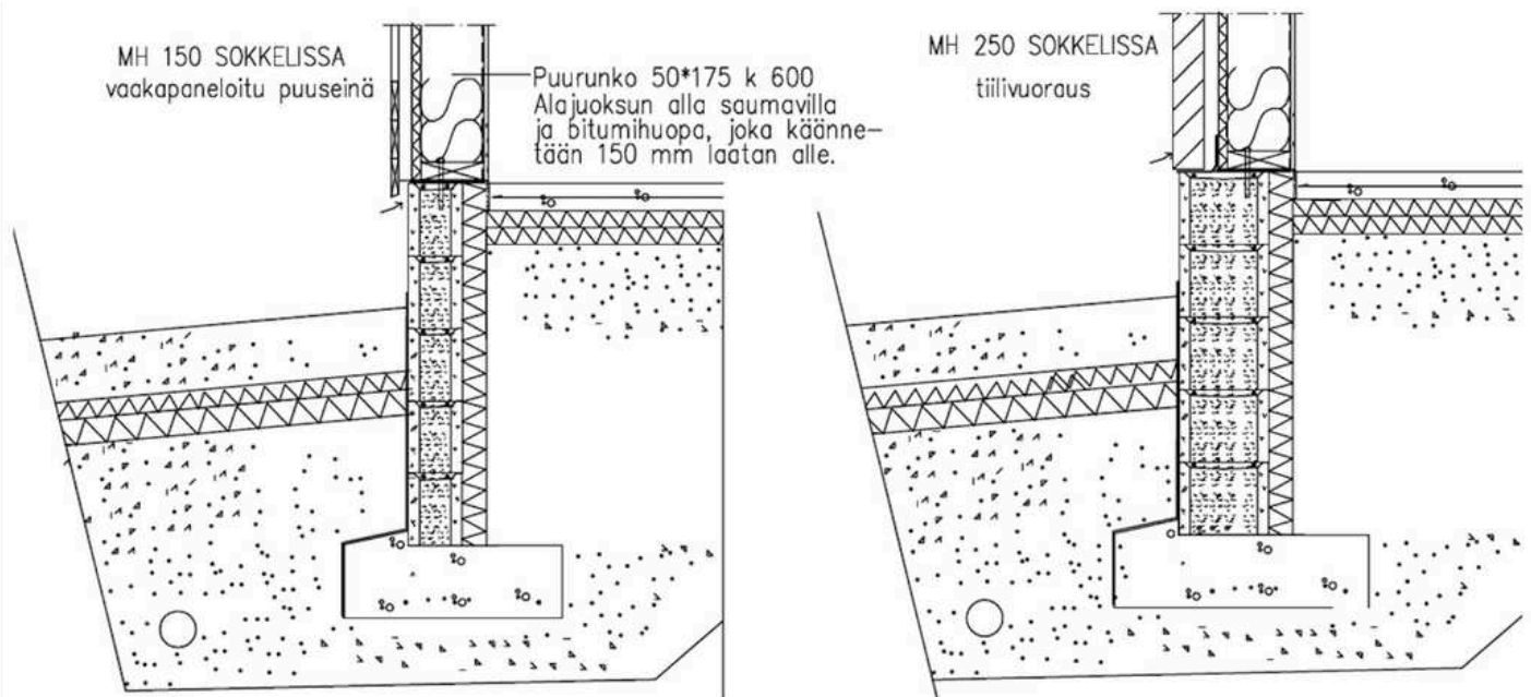
Kuva 15. Esimerkki sokkeliratkaisuista.
