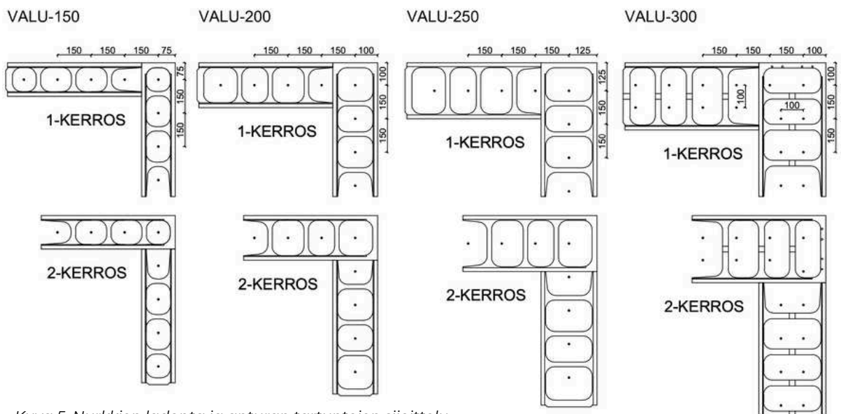
Kuva 5. Nurkkien ladonta ja anturan tartuntojen sijoittelu.
