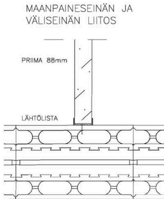
Kuva 11. Maanpaineseinän ja HB-Priima väliseinäharkon liitos lähtölistalla.
