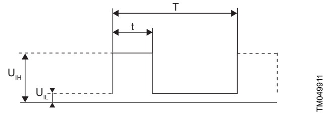
PWM-signaali
