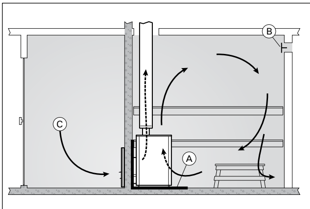
Figuur 6. Afzuiging door zwaartekracht
