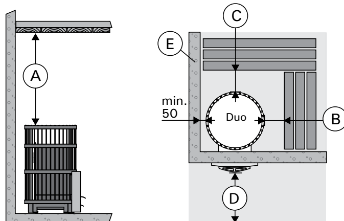
Figure 9. Distanze di sicurezza (tutte le dimensioni sono fornite in millimetri) Figura 9. Distanze di sicurezza (tutte le dimensioni sono espresse in millimetri)
