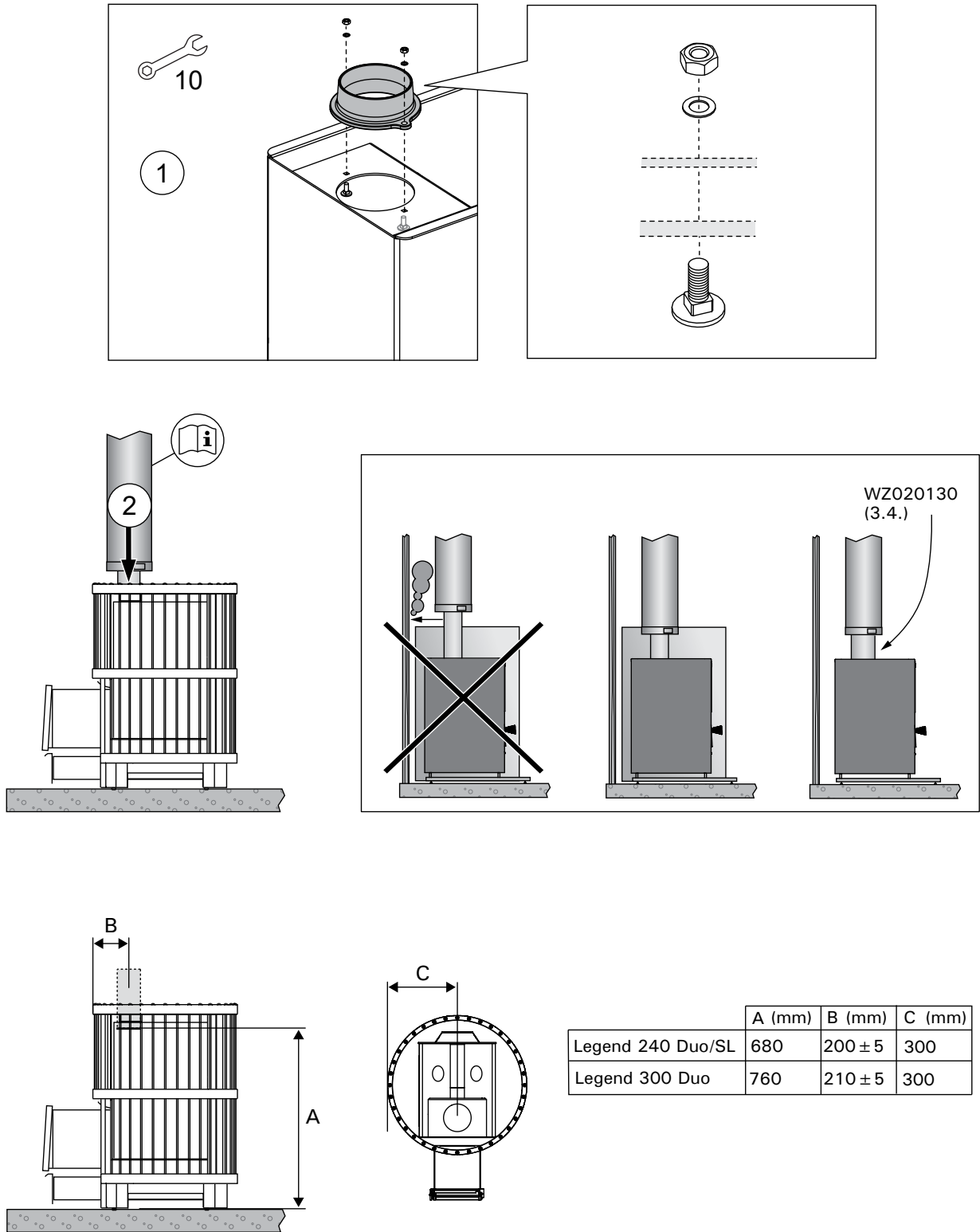
Kuva 11. Kiukaan liittäminen Harvia-teräspiippuun Bild 11. Anslutning av ugnen till Harvia stålkorsten
