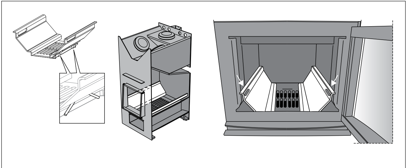
Figure 2. Combustion air channels Abbildung 2. Verbrennungsluftkanäle
