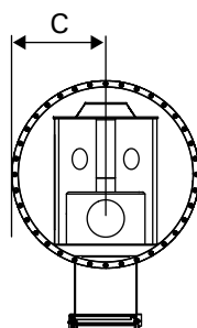
Рисунок 11. Присоединение печи к стальному дымоходу Harvia Joonis 11. Kõrse ühendamine Harvia teraskorstnaga
