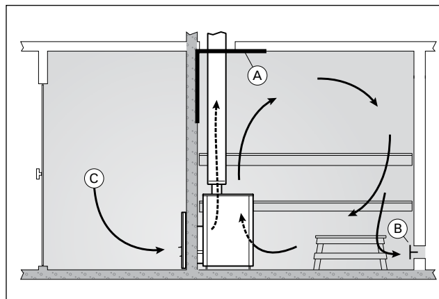
Kuva 7. Koneellinen ilmanvaihto Bild 7. Maskinell ventilation
