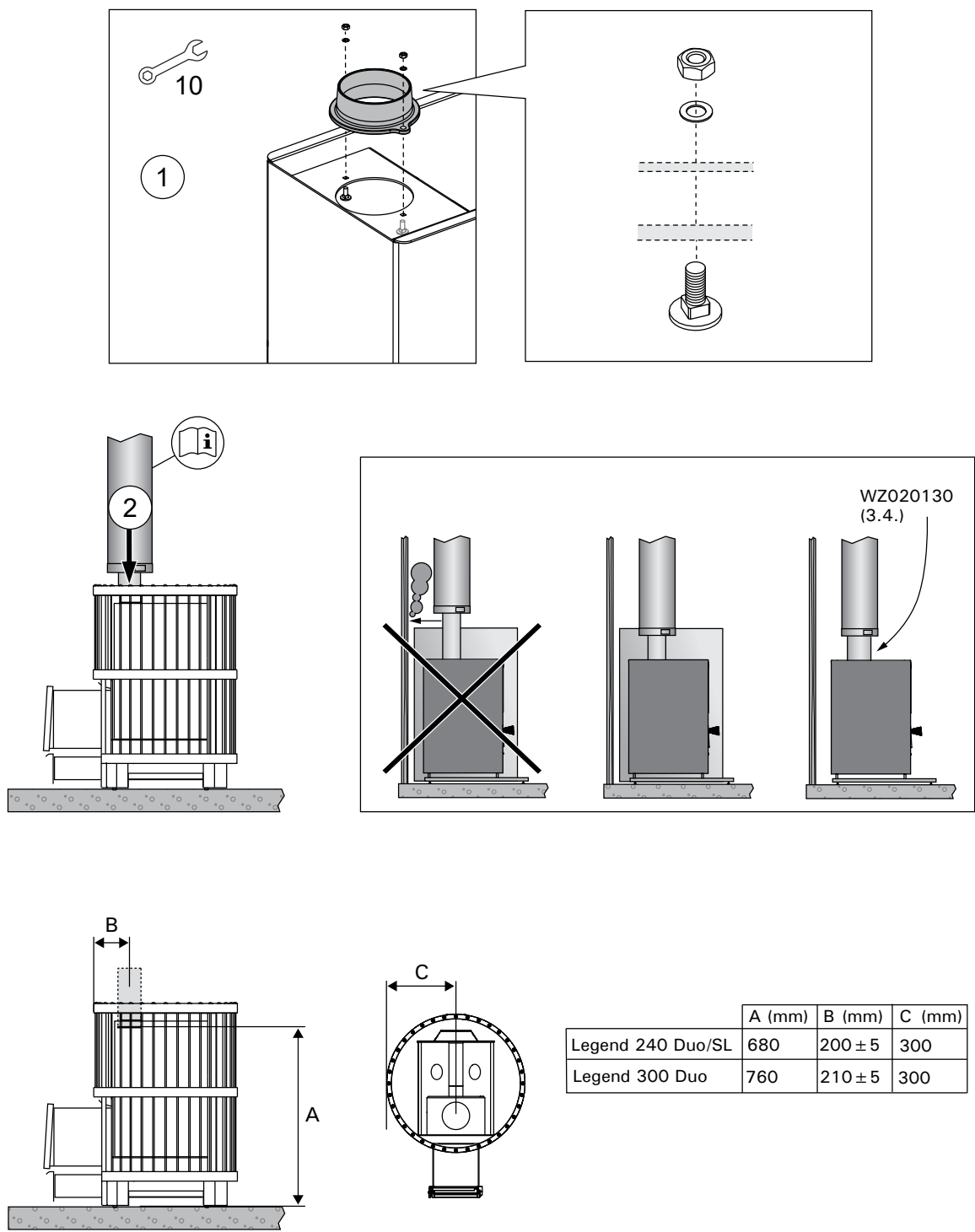
Figuur 11. De kachel aansluiten op een stalen schoorsteen van Harvia
