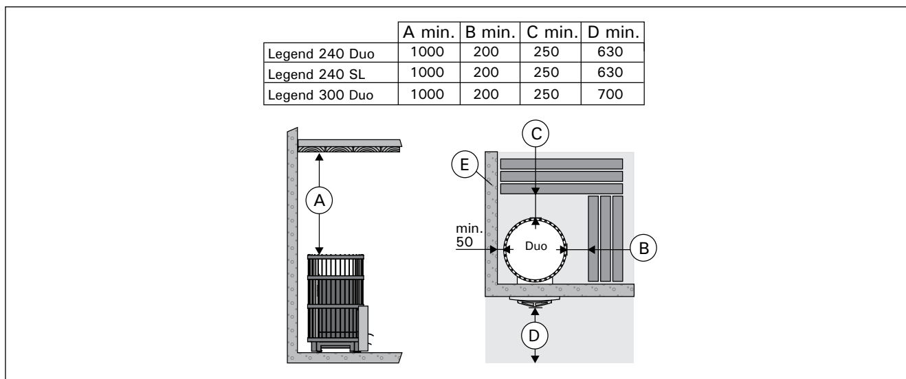
Figuur 9. Veiligheidsafstanden (alle afmetingen in millimeters)
