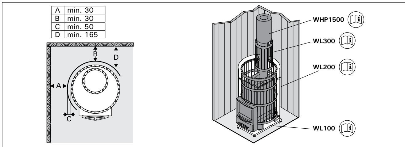
Kuva 10. Legend-suojastarvikkeet (mitat millimetreinä) Bild 10. Legend-skyddstillbehör (mått i millimeter)
