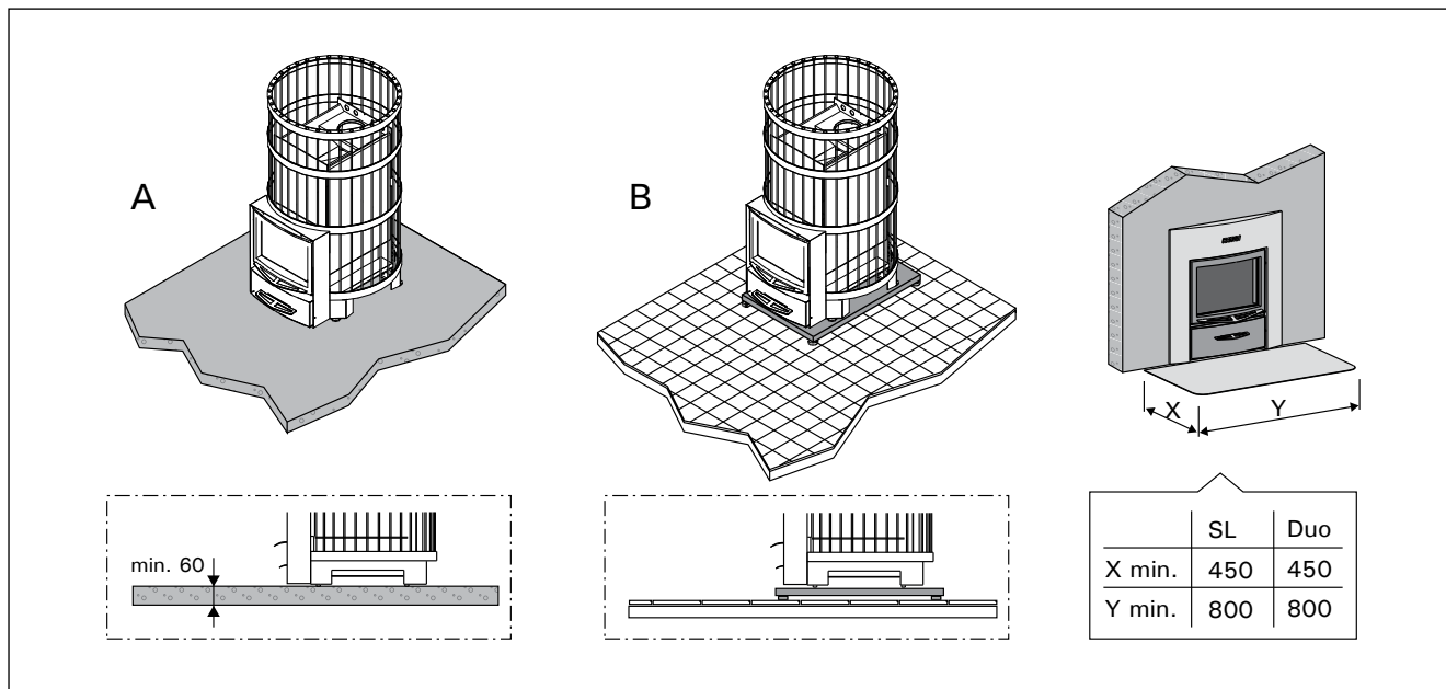
Figure 8. Protection du sol (toutes les dimensions sont fournies en millimètres)
