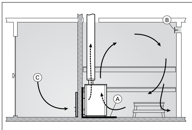
Kuva 6. Painovoimainen ilmanvaihto Bild 6. Självdragsventilation
