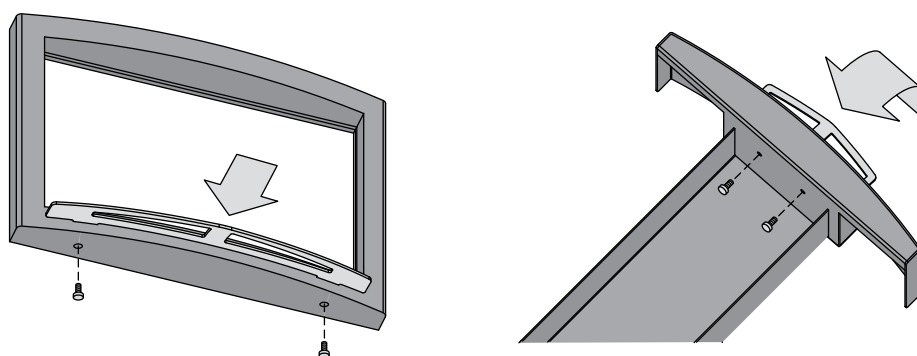
Рисунок 15. Установка рукояток Joonis 15. Käepidemete paigaldamine
