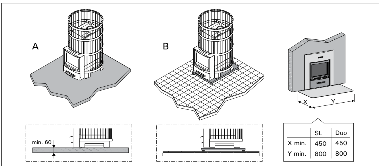
Kuva 8. Lattian suojaaminen (mitat millimetreinä) Bild 8. Skydd av golvet (mått i millimeter)
