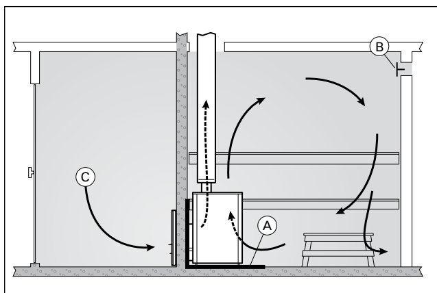
Figure 6. Ventilation par gravité Figura 6. Sistema di ventilazione a gravità
