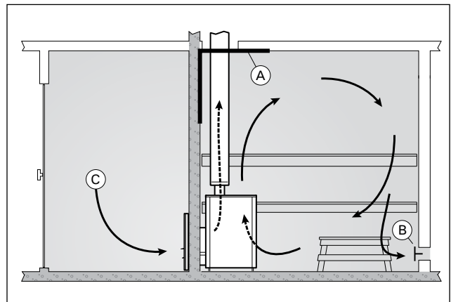
Figuur 7. Mechanische afzuiging
