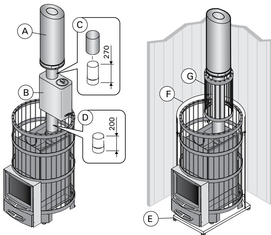
Figuur 15. Accessoires (alle afmetingen in millimeters)
