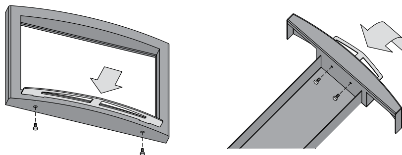
Figuur 15. De handgrepen installeren, Legend 240 Duo, 300 Duo
