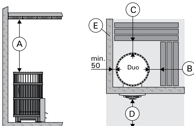
Kuva 9. Suojaetäisyydet (mitat millimetreinä) Bild 9. Säkerhetsavstånd (mått i millimeter)
