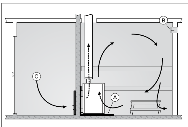
Figure 6. Gravity exhaust ventilation Abbildung 6. Schwerkraftentlüftung
