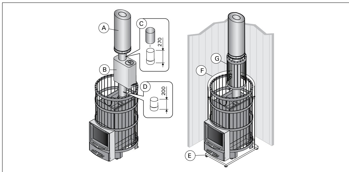
Kuva 16. Lisätarvikkeet (mitat millimetreinä) Bild 16. Tilläggsutrustning (måttan i millimeter)
