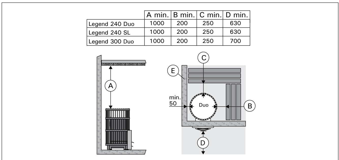
Figure 9. Safety distances (all dimensions in millimeters) Abbildung 9. Sicherheitsabstände (alle Abmessungen in Millimetern)
