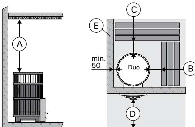
Рисунок 9. Безопасные расстояния (все размеры приведены в миллиметрах)
