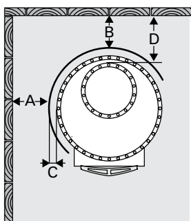
Рисунок 10 Элементы защиты Legend
