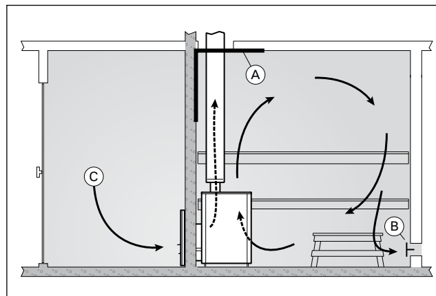
Figure 7. Mechanical exhaust ventilation Abbildung 7. Mechanische Entlüftung
