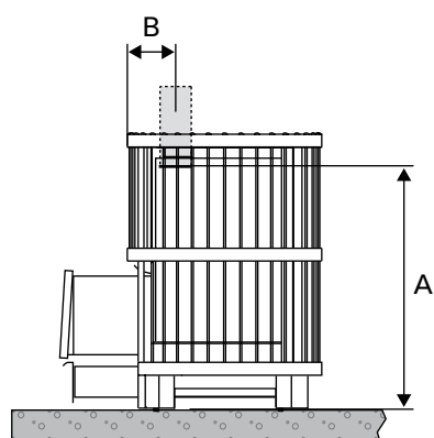
Рисунок 11. Присоединение печи к стальному дымоходу Harvia Joonis 11. Kõrse ühendamine Harvia teraskorstnaga
