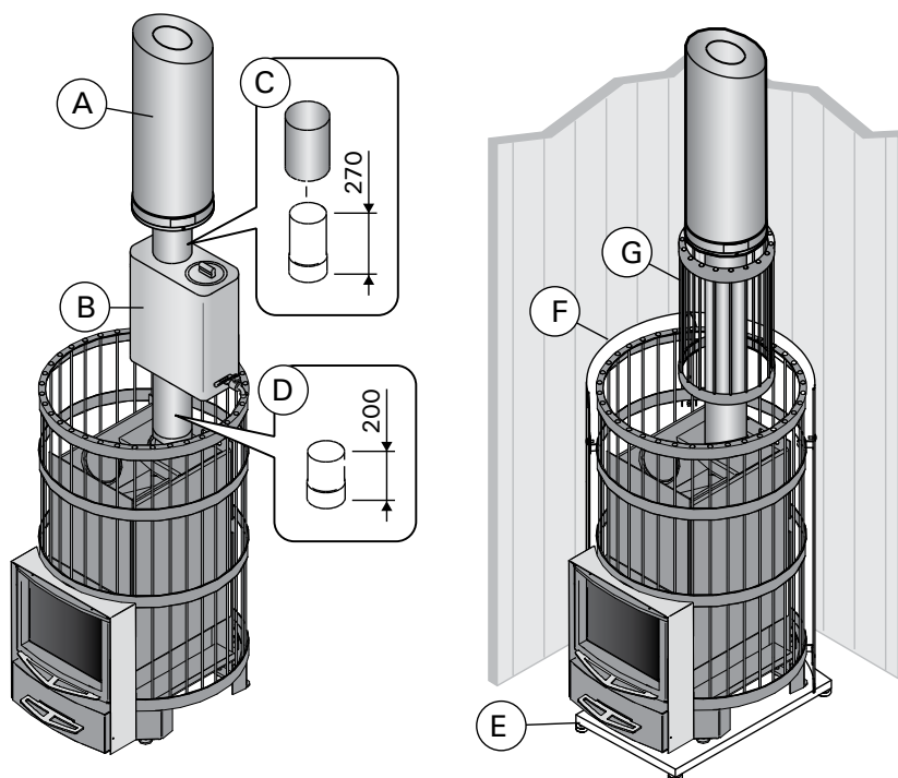
Рисунок 16. Дополнительные принадлежности (все размеры приведены в миллиметрах)
