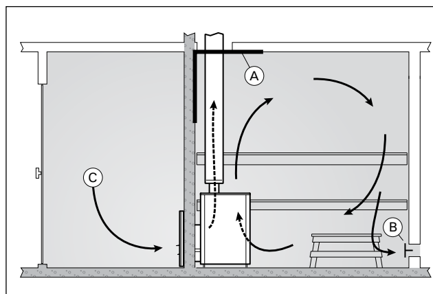
Figure 7. Ventilation mécanique Figura 7. Sistema di ventilazione meccanico
