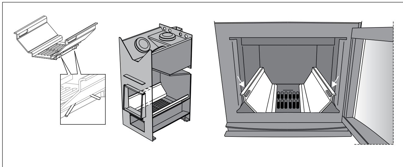
Рисунок 2. Каналы для подачи воздуха для горения Joonis 2. Põlemiskambri õhukanalid
