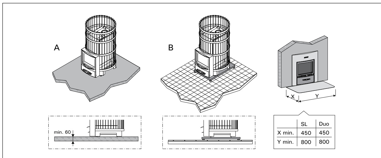
Figuur 8. De vloer beschermen (alle afmetingen in millimeters)
