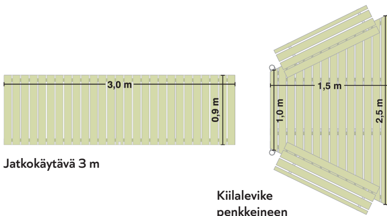
Tarvikelaituri 6 penkillä, 7,6 m
