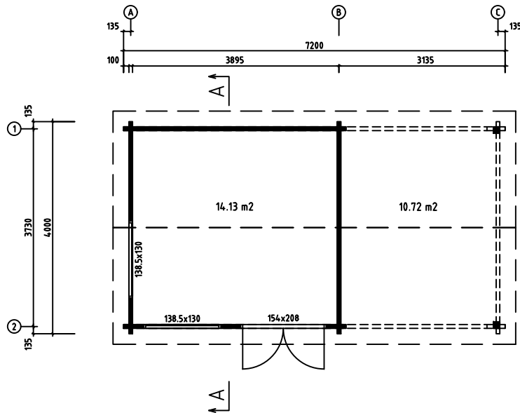
POHJAPIIRUSTUS
