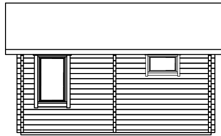
JULKISIVU 4
