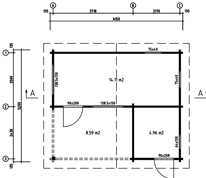
POHJAPIIRUSTUS
