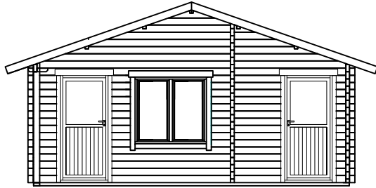
JULKISIVU 2
