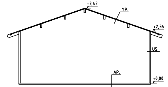
LEIKKAUS A-A
