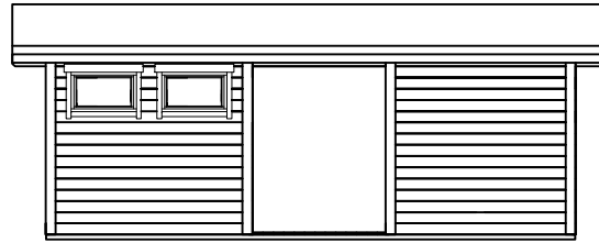
JULKISIVU 4
