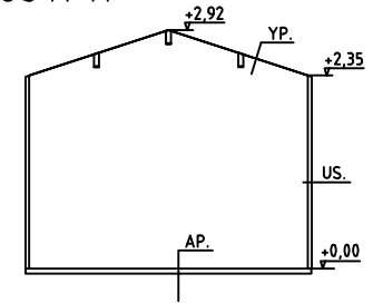
LEIKKAUS A-A
