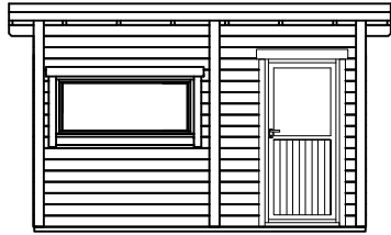
JULKISIVU 2
