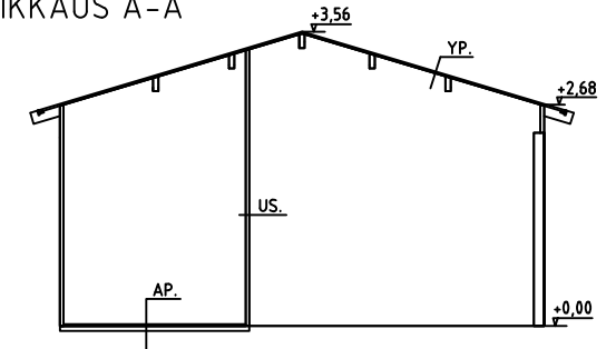
LEIKKAUS A-A
