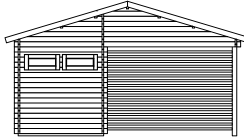
JULKISIVU 4
