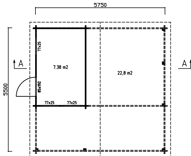
POHJAPIIRUSTUS
