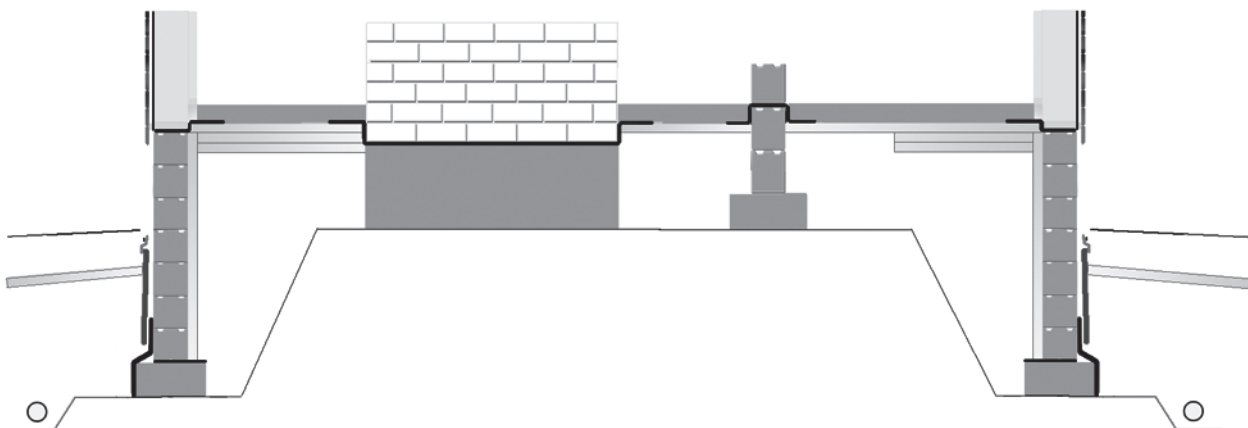
Koko pohja.
