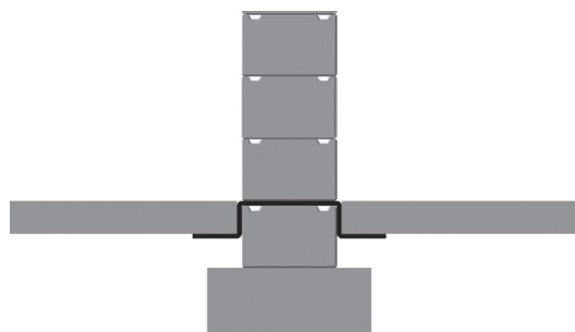
Kantava väliseinä.
